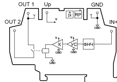
Рис. 5.2 Схема расположения клемм в корпусе преобразователя
