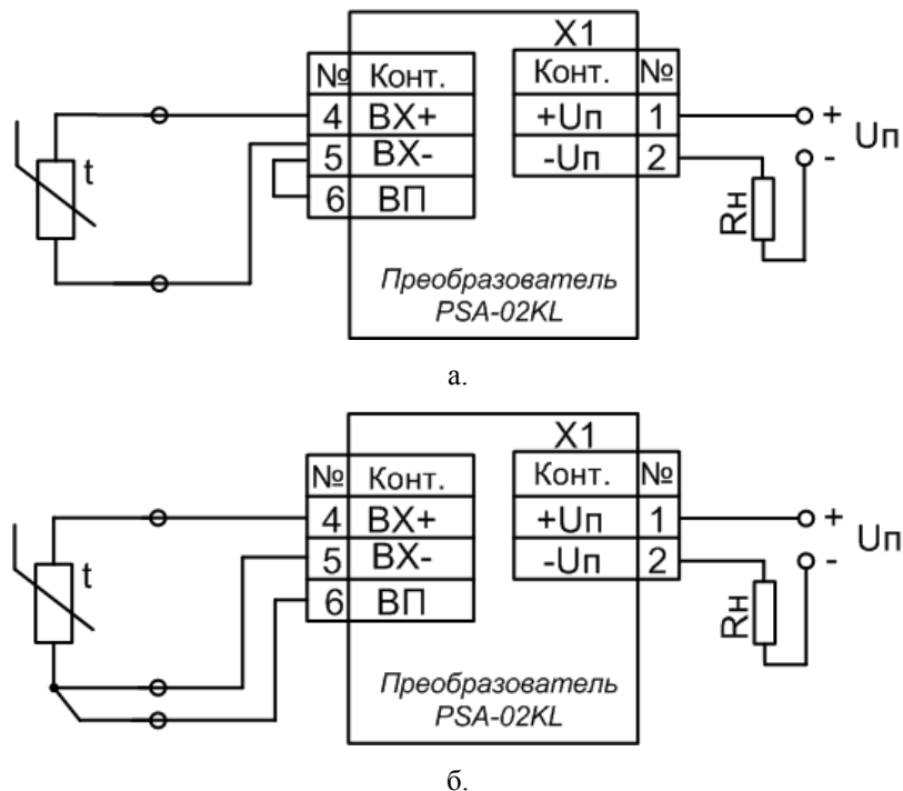
Рис. 4.1 Схема подключения преобразователя. а) датчик термосопротивления с двухпроводной схемой подключения; б) датчик термосопротивления с трехпроводной схемой подключения
